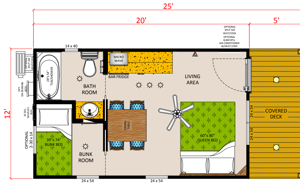
CABANA/KOA 20FP (240 SQ.FT.)+(DECK)
