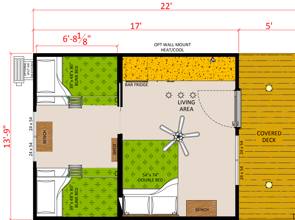
CLOVERDALE/KOA 22FP (234 SQ.FT.)+(DECK)
